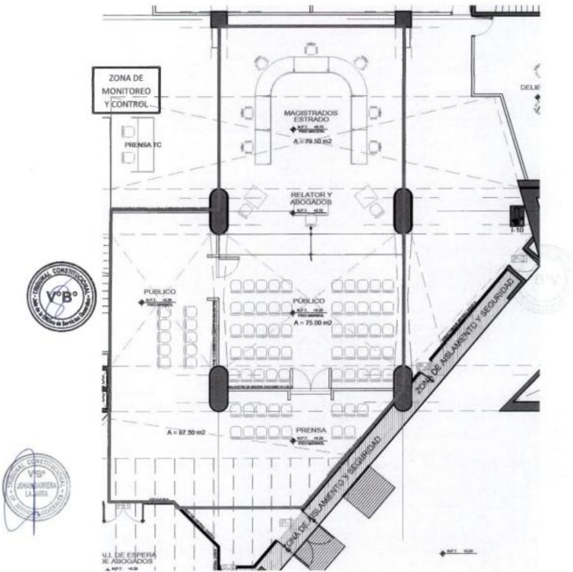
Planta de distribución Sala de Audiencias, Sede San Isidro
